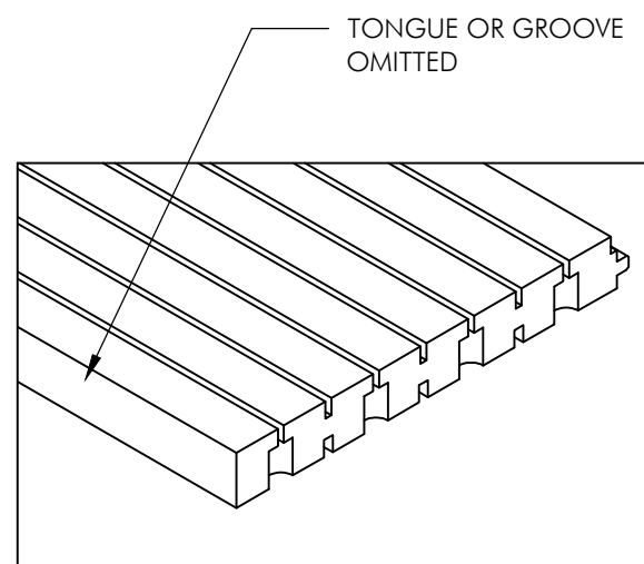
FINISHED LONGITUDINAL EDGE*
